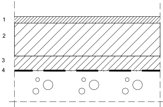
Rakenneleikkaus 1:1
